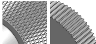
널링
